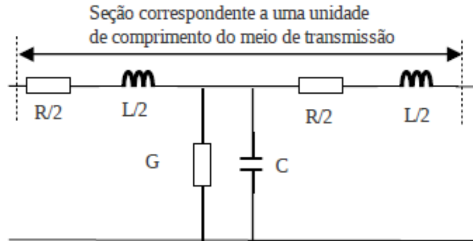
Figura 29: Modelo elétrico da linha de transmissão
