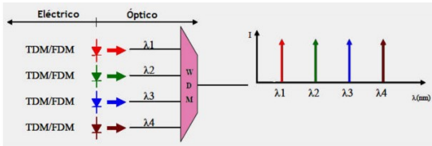
Multiplexagem WDM
