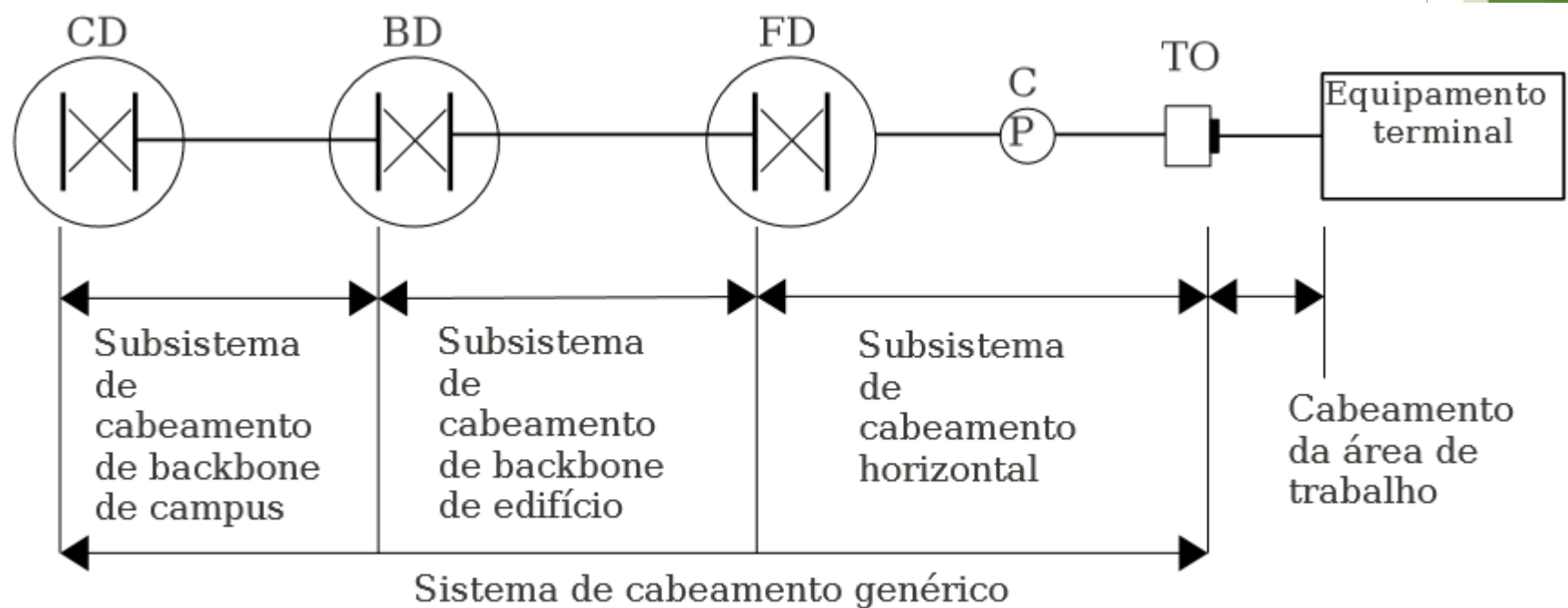
Figura 11: Estrutura do cabeamento genérico
