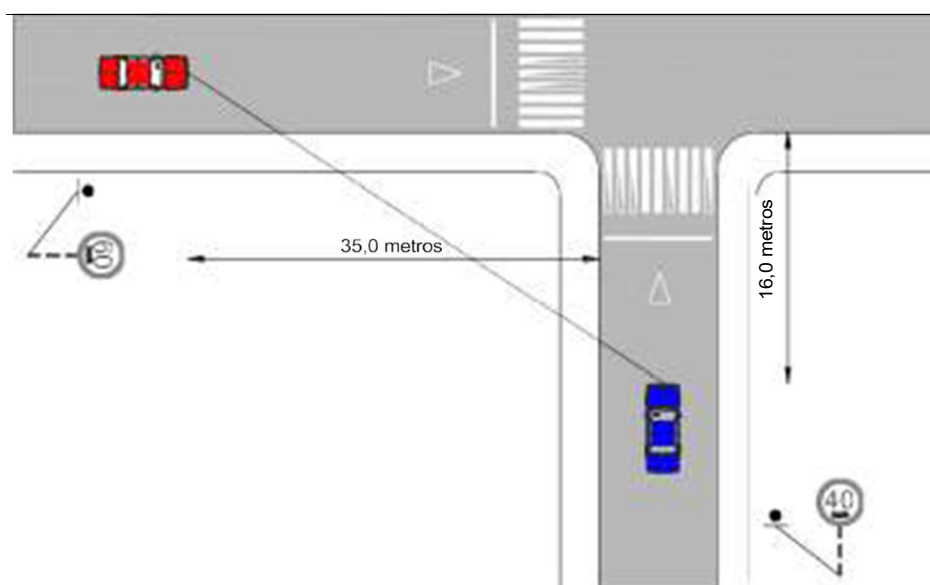
Figura 3.20: Interseção em "T", de vias com velocidades regulamentadas de 60 km/h e 40km/h
