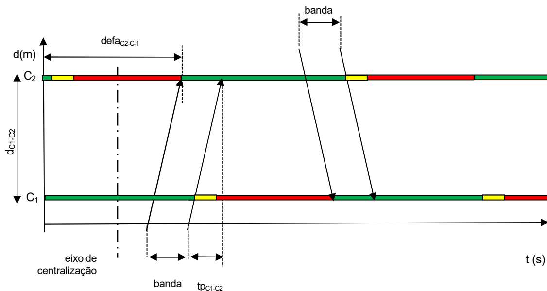
Figura 9.8: Exemplo de coordenação em via de mão dupla com verde e vermelho centralizados
