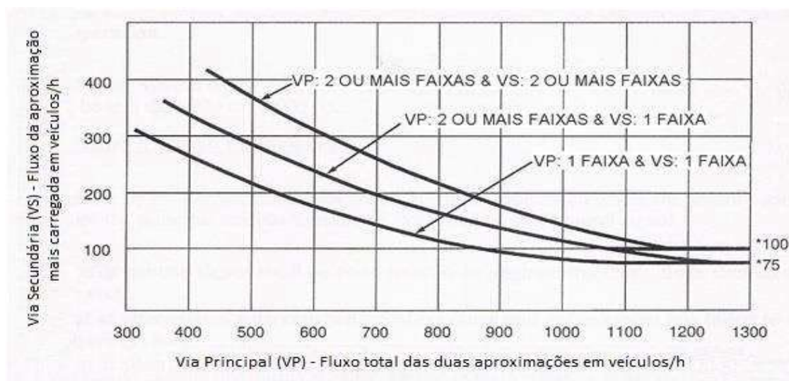
Figura 3.16: Valores de volume (fluxo) que justificam a implantação de sinalização semafórica em locais em fase de projeto: Caso 2 (Fonte: MUTCD-2003)
