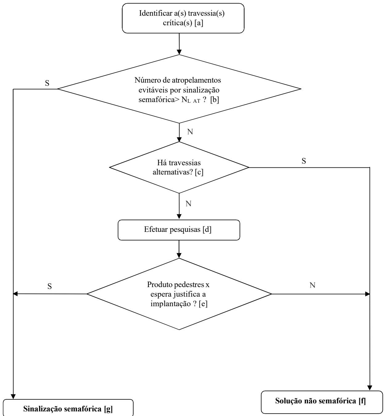
Figura 3.10: Estudos em locais existentes: abordagem pedestres
