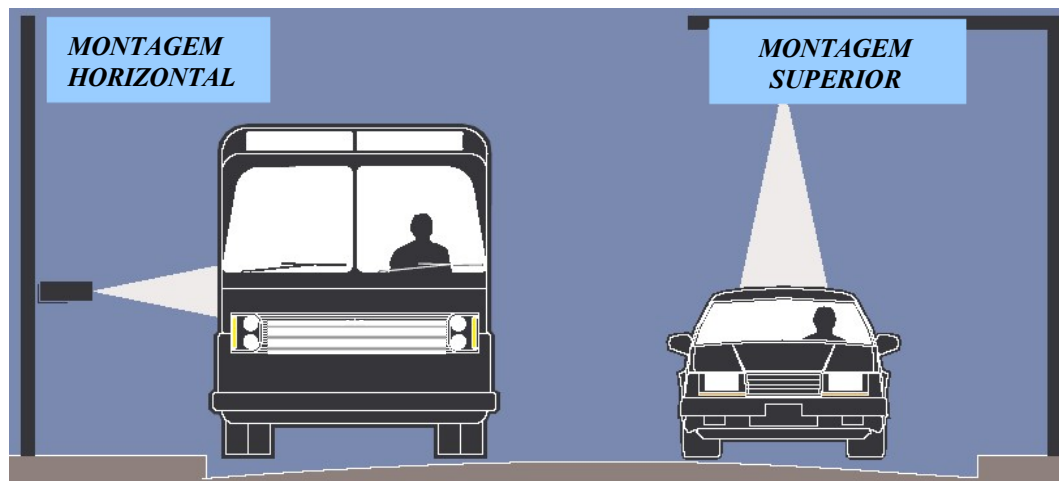
Figura 2.13: Formas de posicionamento dos detectores ultrassônicos
