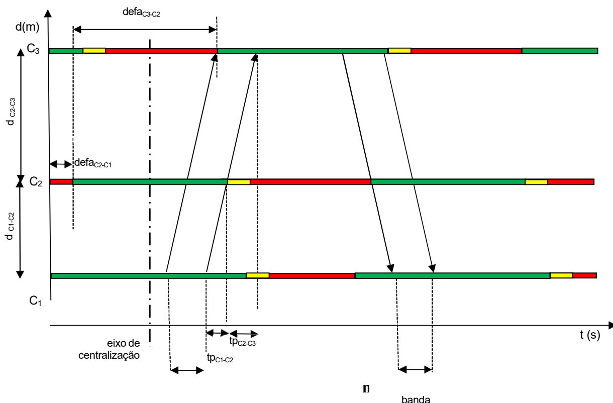
Figura 9.9: Exemplo de coordenação e coordenação em via de mão dupla com combinação de estratégias
