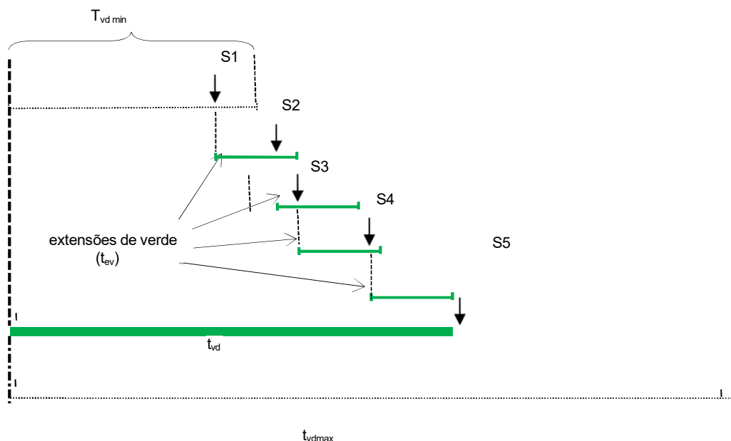
Figura 8.1: Funcionamento de um estágio atuado em função de solicitações de veículos
