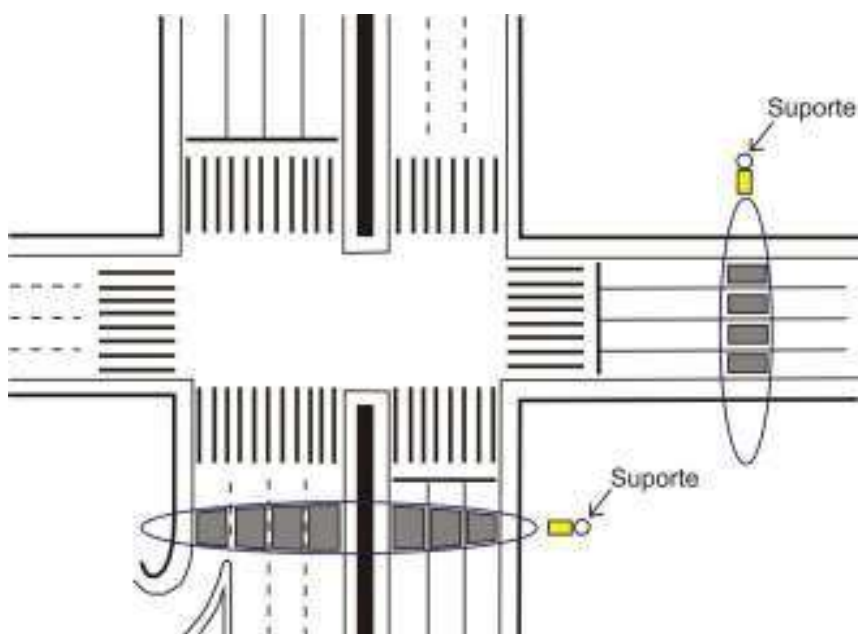
Figura 2.10: Ilustração da configuração transversal de detectores por microondas
