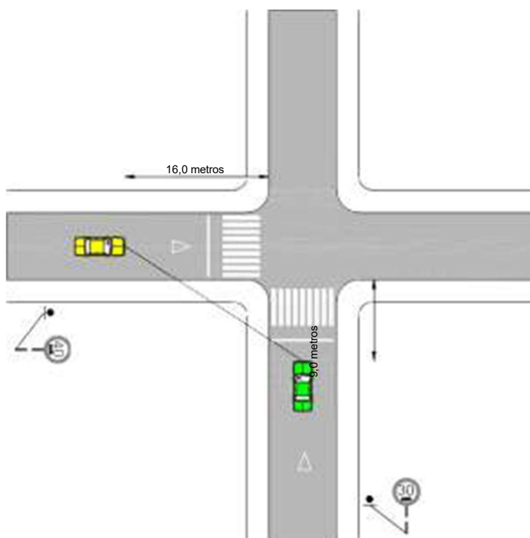
Figura 3.19: Interseção de vias com velocidades regulamentadas de 40 km/h e 30 km/h
