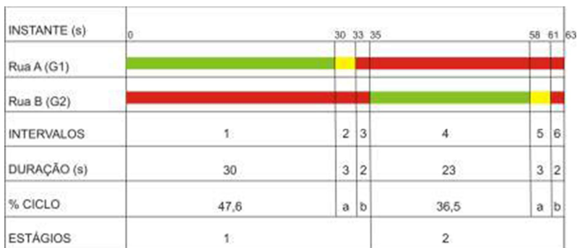
Figura 7.10: Diagrama de intervalos luminosos para o tempo de ciclo de 63s
