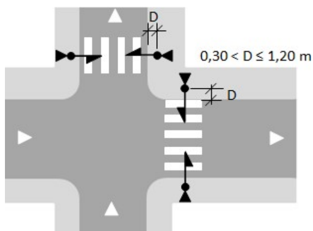
Figura 10.14: Afastamento da botaieira com relação ao meio-fio
