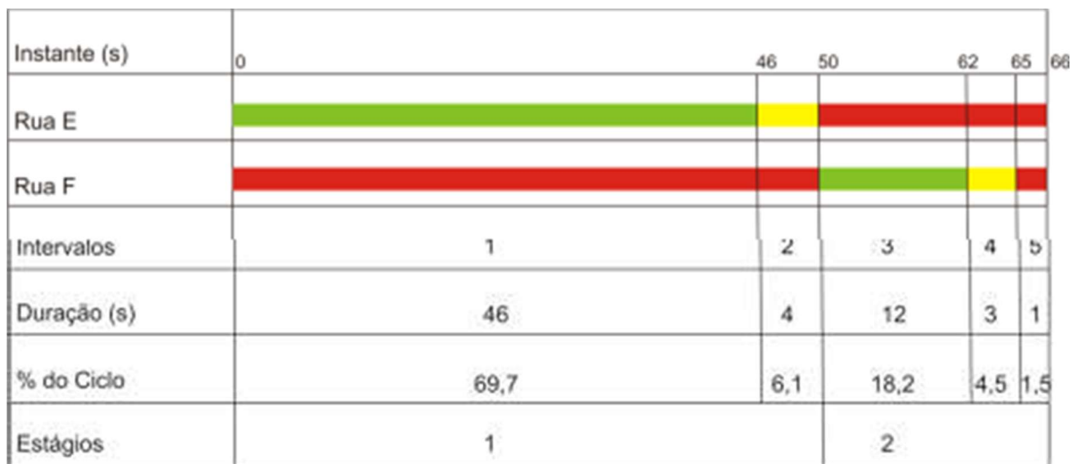
Figura 7.21: Diagrama dos intervalos luminosos para o tempo de ciclo de 66s
