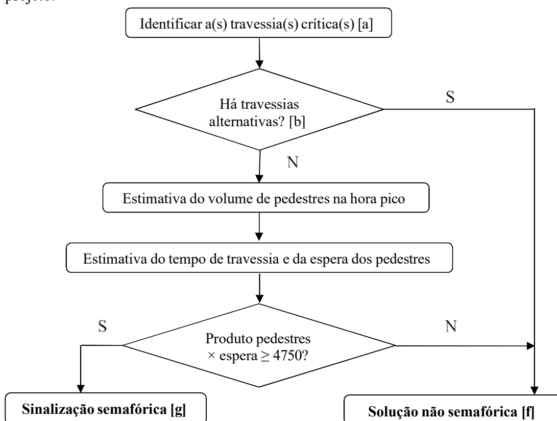
Figura 3.13: Estudos em locais em fase de projeto: abordagem pedestres
