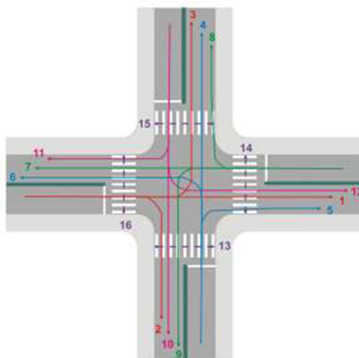
Figura 3.7: Exemplo de um diagrama de conflitos
