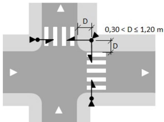
Figura 10.15: Boteeira única para atender duas travessias
