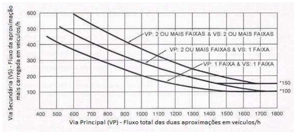
Figura 3.15: Valores de volume (fluxo) que justificam a implantação de sinalização semafórica em locais em fase de projeto: Caso 1 (Fonte: MUTCD-2003)
