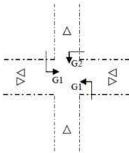
Figura 8.7: Distribuição dos grupos semaforicos
