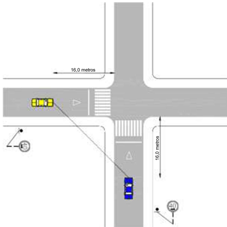
Figura 3.17: Interseção de duas vias com velocidade regulamentada de 40 km/h
