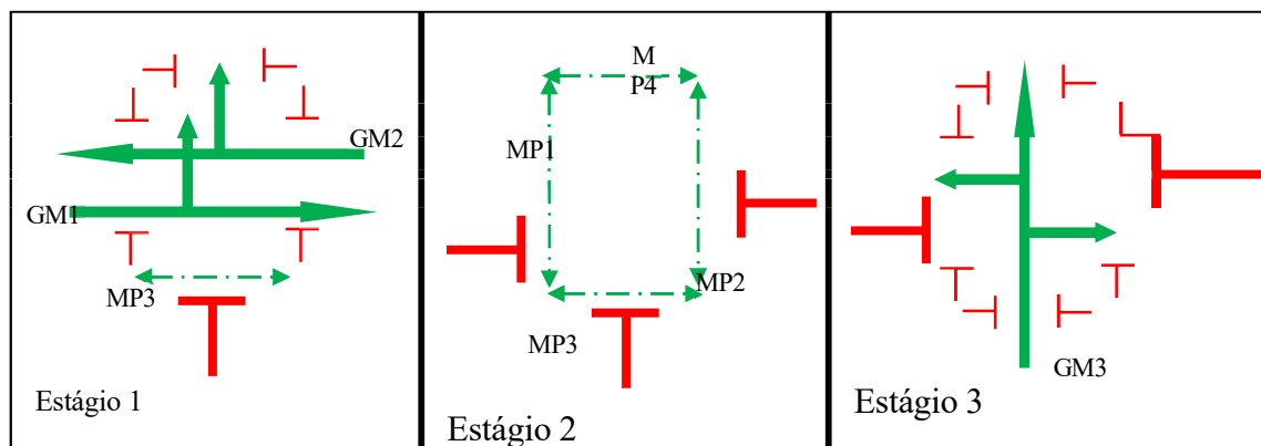
Figura 7.25: Diagrama de estágios
