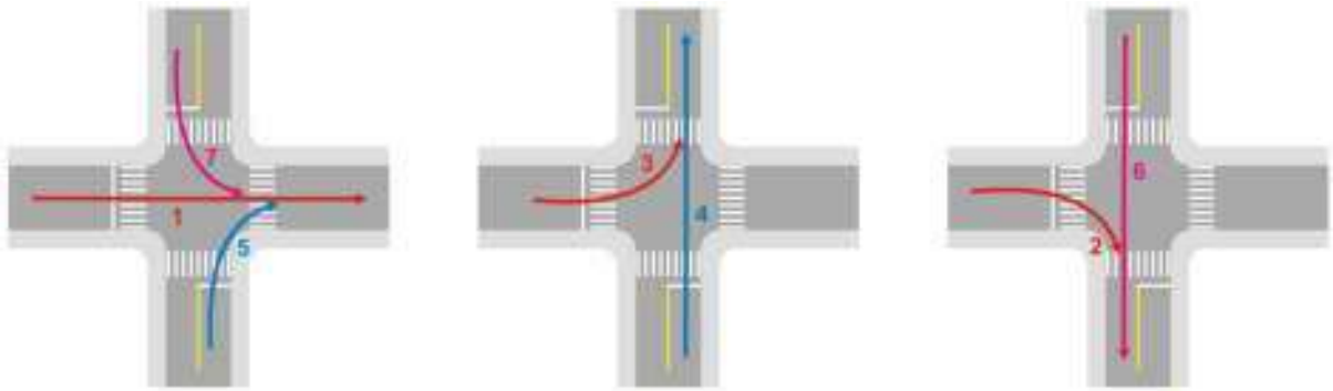
Figura 3.3: Movimentos convergentes
