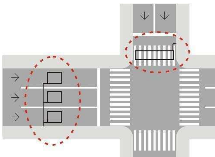
Figura 2.5: Exemplo de laços indutivos empregados para detecção veicular
