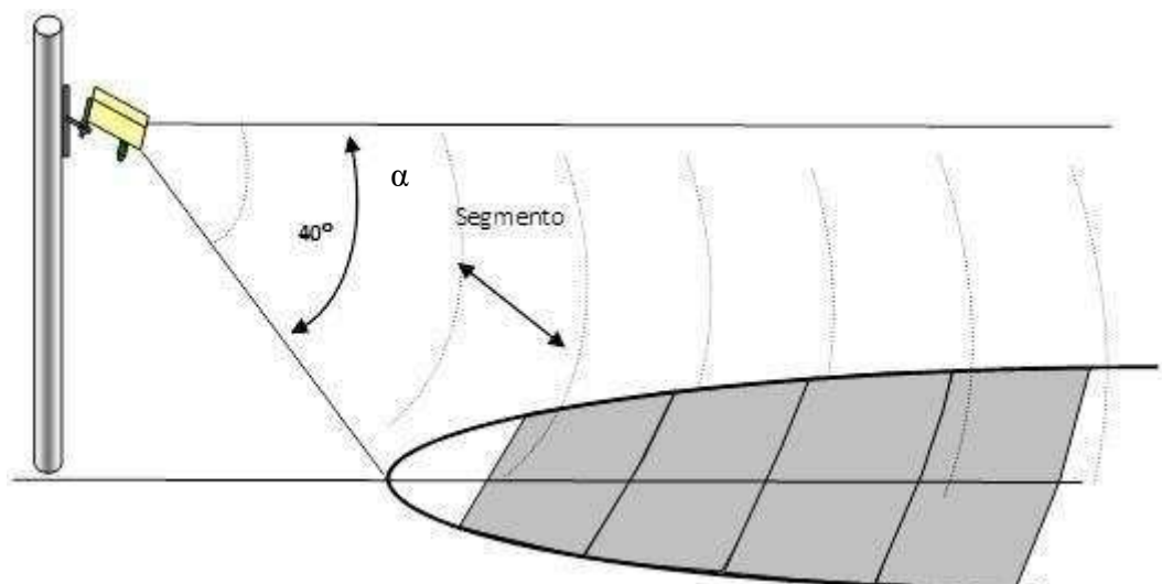
Figura 2.9: Feixe de microondas do RTMS e sua superfície oval
