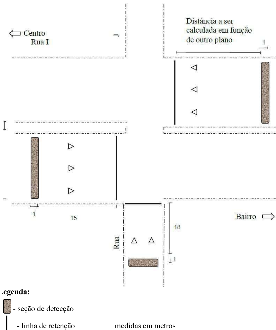
Figura 8.8: Posicionamento das seções de detecção
