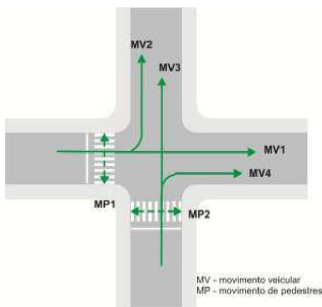
Figura 3.1: Representação de movimentos em uma interseção de duas vias de mão única
