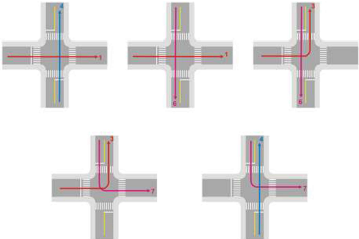
Figura 3.5: Movimentos interceptantes
