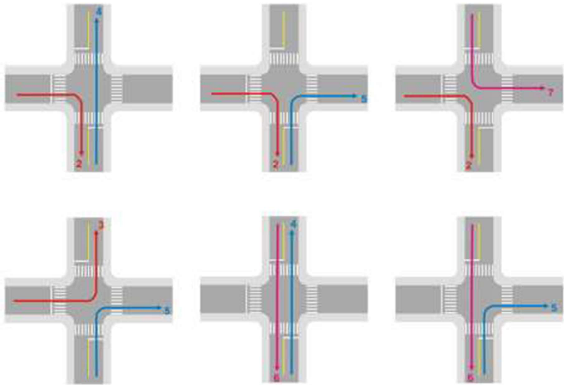
Figura 3.6: Movimentos não-interceptantes
