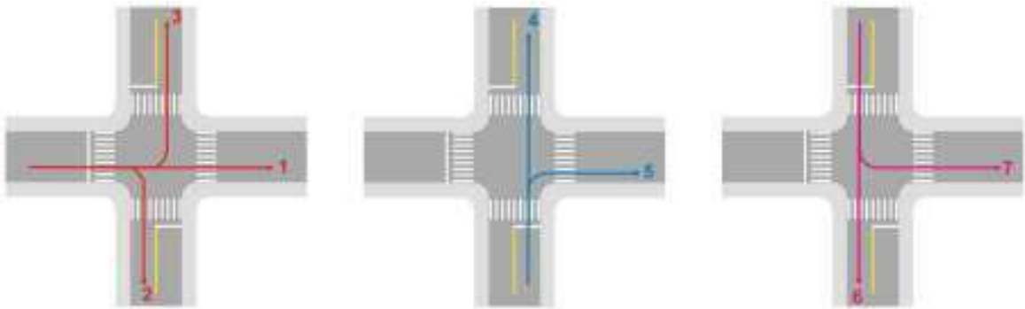
Figura 3.4: Movimentos divergentes
