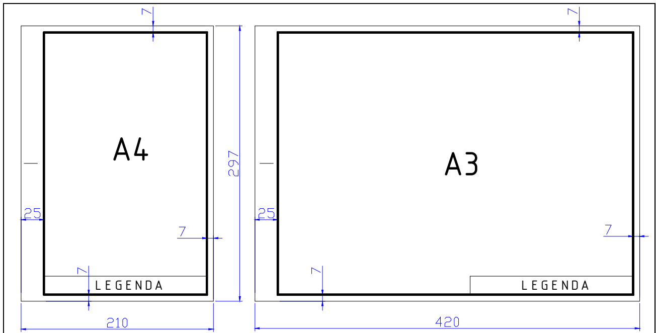
Figura 10.3: Desenho das margens das folhas A4 e A3.
